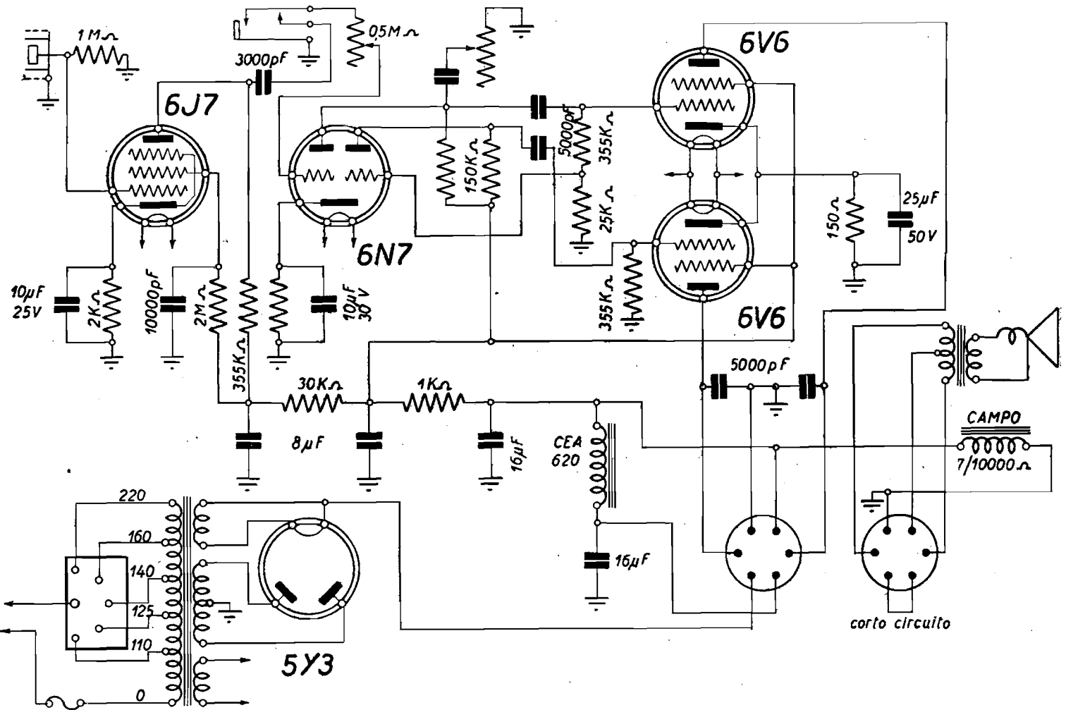
COMPAGNIA GENERALE DI ELETTRICITÀ - Amplificatore da 18 watt.
